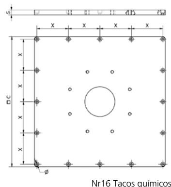
PLACA Z2
