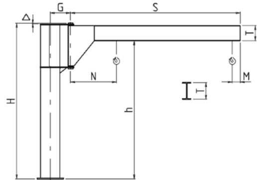
Grúa de columna - Rotación 290°
